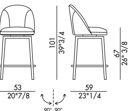
MINNI STOOL_4 gambe metallo / 4 metal legs Design Nello Palomba, Antoy Filips
