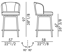
GINGER STOOL_4 gambe metallo / 4 metal legs Design Nello Palomba, Antoy Filips
